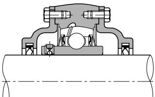
Рис. 2.3. Чугунная крышка
