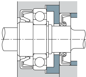
Рис. 11.8. Пример применения масляного уплотнения (1)
