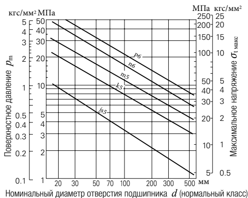
Рис.15.5. Поверхностное давление p_m , а также максимальное напряжение \sigma_{1\text{ макс}} для среднего натяга
