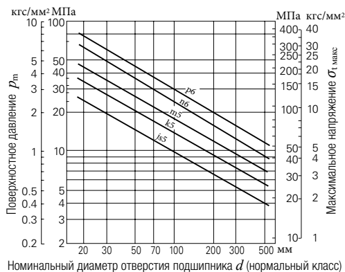
Рис.15.6. Поверхностное давление p_m , а также максимальное напряжение \sigma_{1\text{ макс}} для максимального натяга
