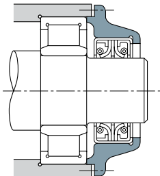
Рис.11.9. Пример применения масляного уплотнения (2)
