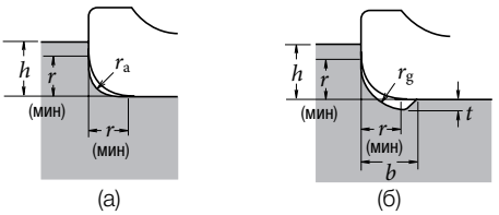
Рис. 11.2. Размеры фасок, радиуса галтели и высоты заплечиков
