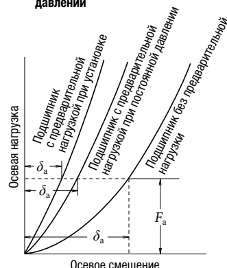
Рис. 10.6. Сравнение жесткости и методов предварительной нагрузки
