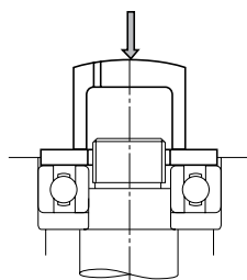
Рис. 14.2. Одновременная запрессовка внутреннего и внешнего колец
