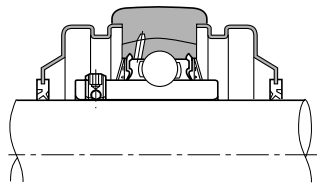
Рис. 2.2. Крышка из штампованной стали
