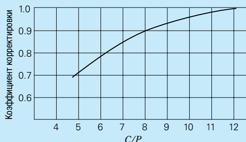
Рис. 6.1. Коэффициент корректировки предельной скорости в зависимости от отношения C/P .
