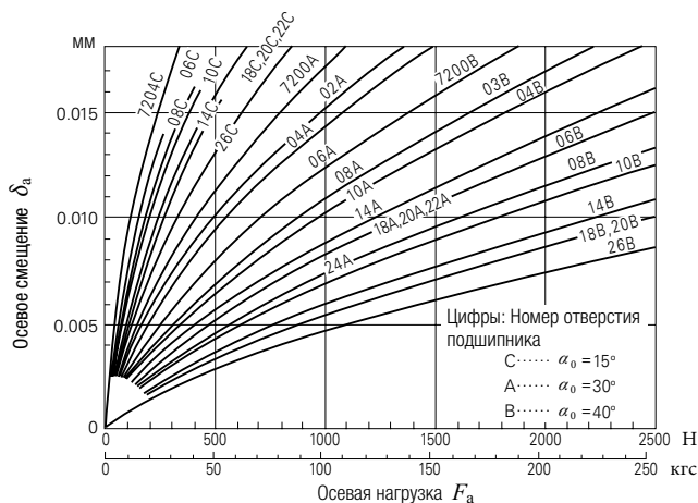
Рис. 15.3. Осевая нагрузка и осевое смещение радиально-упорных шарикоподшипников
