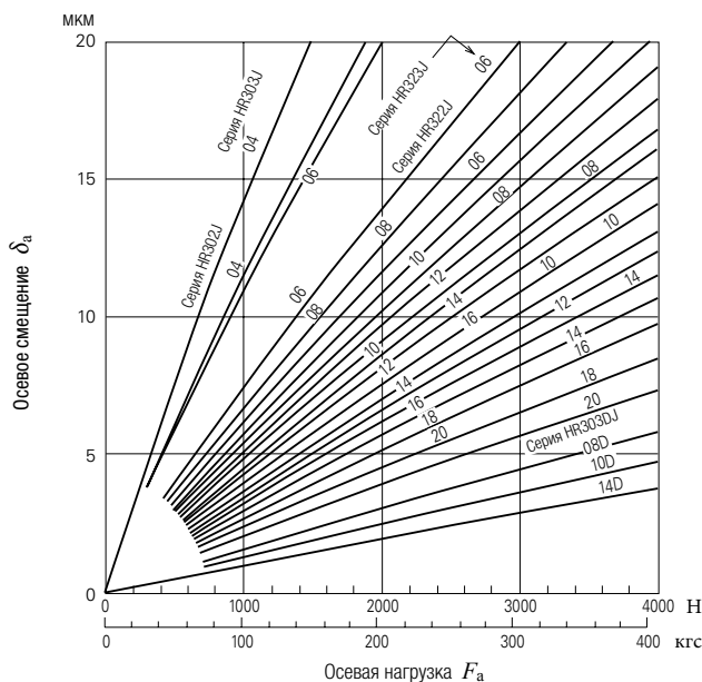
Рис. 15.4. Осевая нагрузка и осевое смещение конических роликоподшипников
