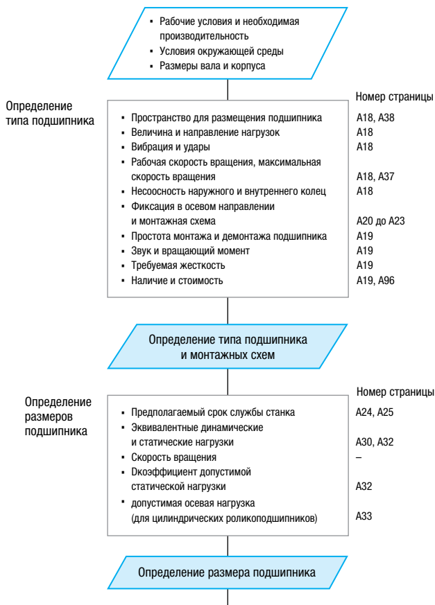
Рисунок 2.1. Схема подбора подшипников качения
