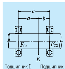
Рисунок 5.5. Распределение радиальной нагрузки (1)
