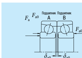
Рис.10.3. Предварительный натяг дуплексных подшипников, установленных по схеме «спина к спине».
