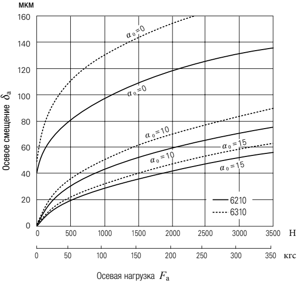
Рис. 15.2. Осовая нагрузка и осевое смещение радиальных шарикоподшипников
